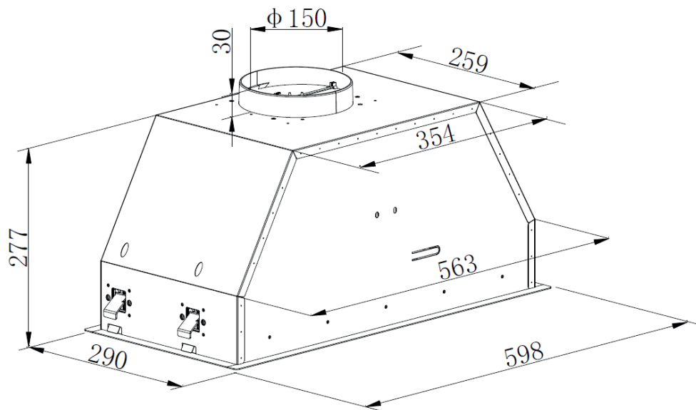
Рис. 1 Внешний вид кухонной вытяжки и схема размеров
